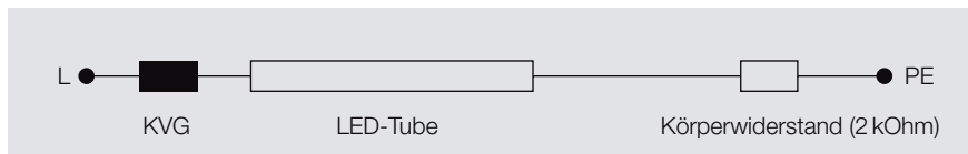
Möglicher Körperstrom von 20 bis 90 mA bei einseitigem Einführen/Einrasten einer LED-Röhre.
